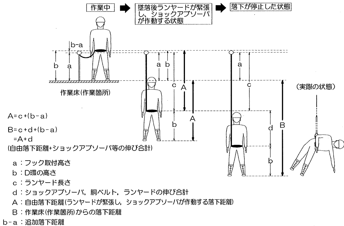
図2 胴ベルト型の落下距離等
